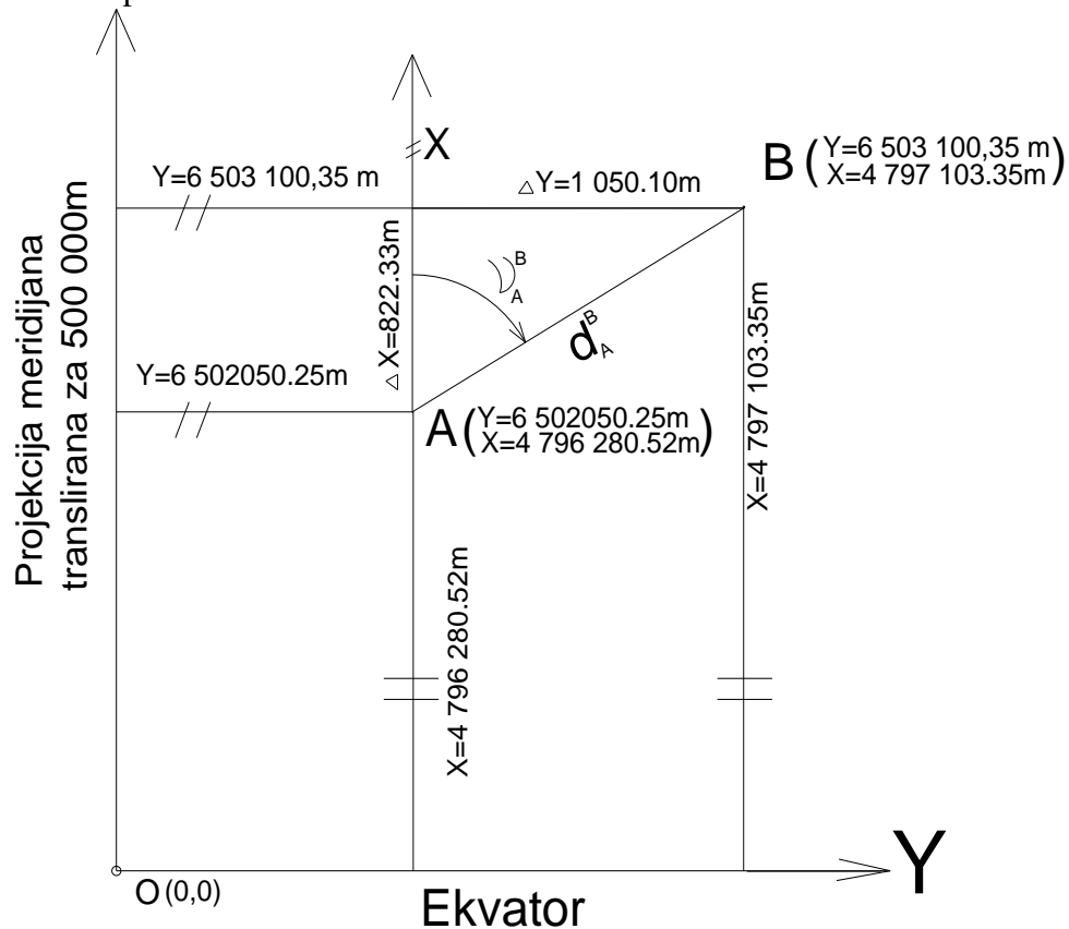
Slika 4. Direkcioni ugao
