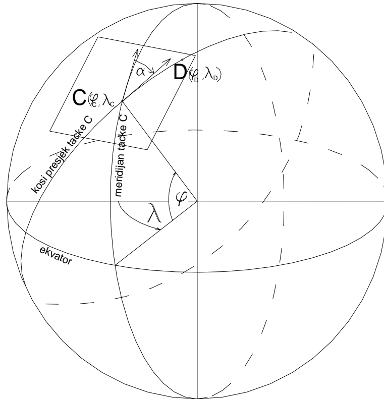
Slika 2. Geodetski azimut
